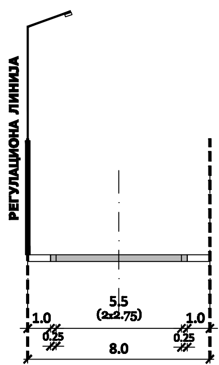
ПОПРЕЧНИ ПРОФИЛ 1-1
