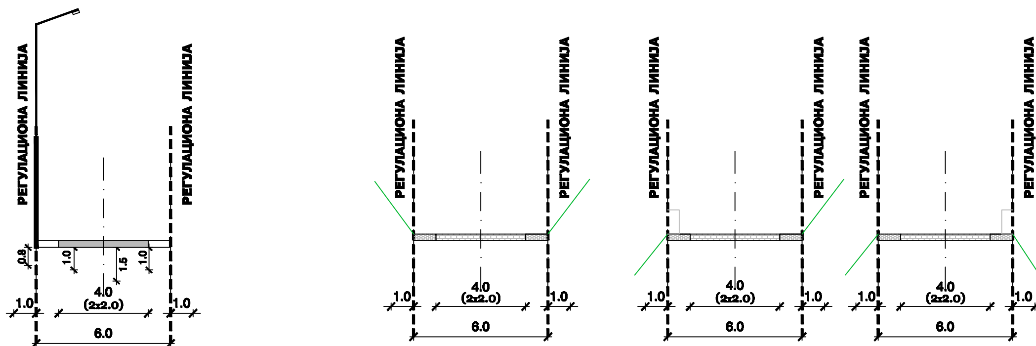
ПОПРЕЧНИ ПРОФИЛ 2-2
